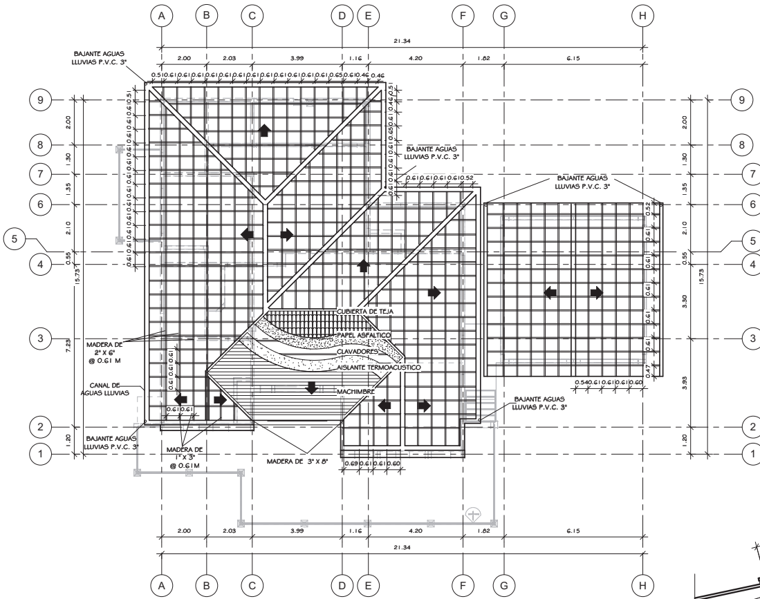
PLANTA ESTRUCTURAL DE TECHOS
