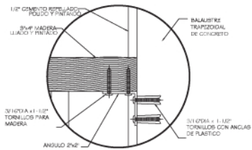
DETALLE ANCLA DE PASAMANO A BALAUSTR
