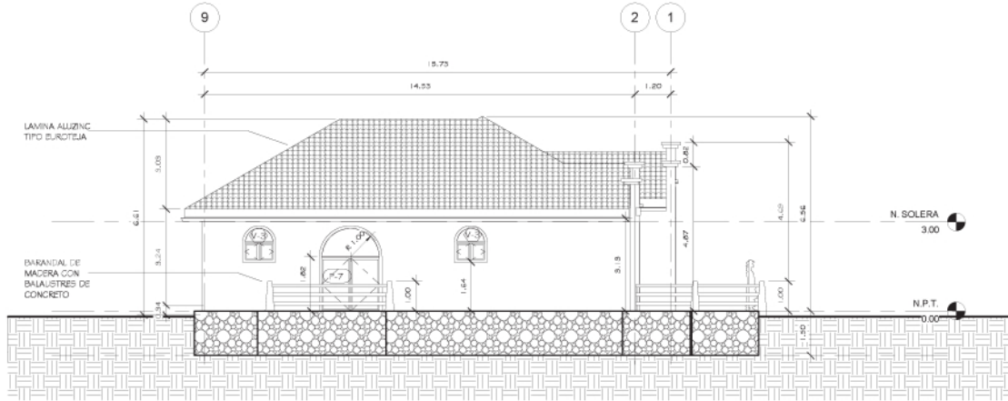
ELEVACION DERECHA
