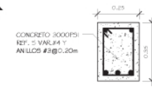
SECCION T. DE VIGA VI-2
