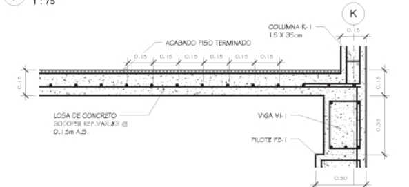
SECCION ESTRUCTURAL DE LOSA MONOLITICA
