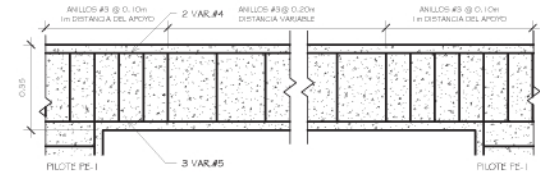
SECCION L. DE VIGA VI-1
