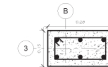
SECCION DE CASTILLO C-3
