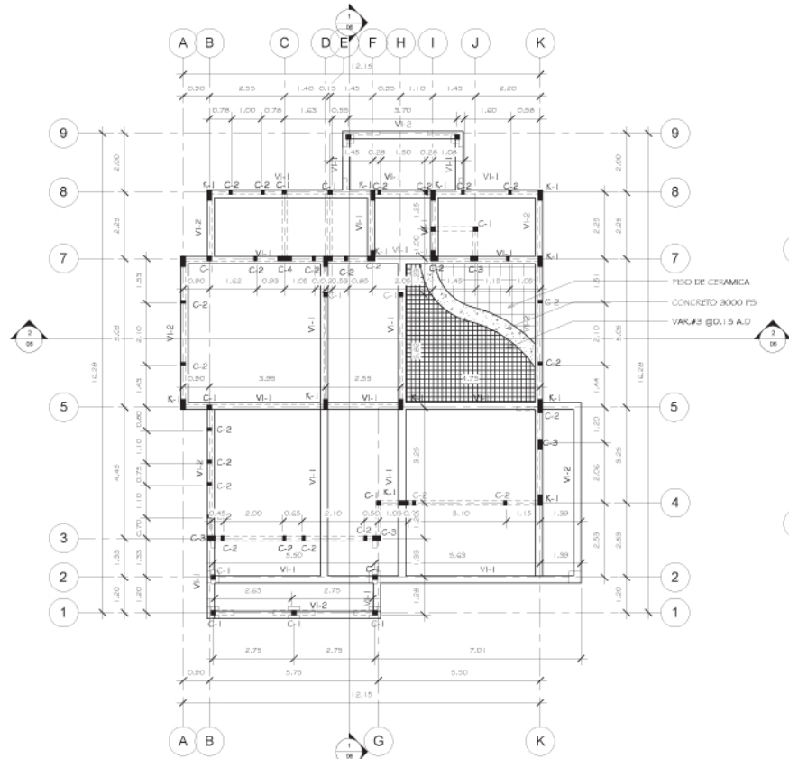
PLANTA ESTRUCTURAL ENTREPISO NIVEL I
