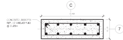
SECCION DE CASTILLO C-4
