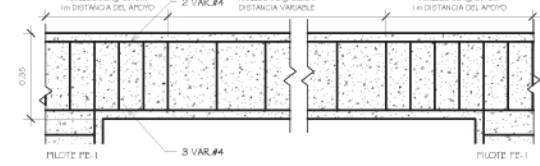
SECCION L. DE VIGA VI-2
