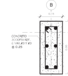
SECCION DE COLUMNA K-1
