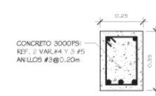
SECCION T. DE VIGA VI-1
