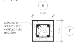
SECCION DE CASTILLO C-1
