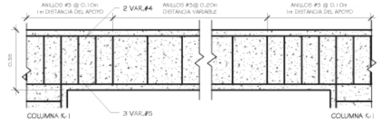
SECCION L. DE VIGA VI-1 (NIVEL2)
