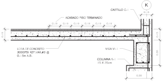
SECCION ESTRUCTURAL DE LOSA MONOLITICA(NIVEL2)
