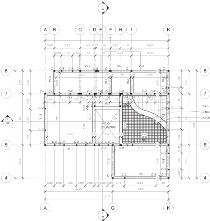
PLANTA ESTRUCTURAL DE ENTREPISO NIVEL 2
