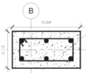
SECCION DE CASTILLO C-3(NIVEL2)
