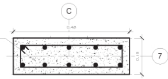
SECCION DE CASTILLO C-4(NIVEL2)
