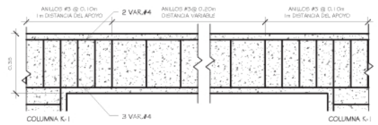
SECCION L. DE VIGA VI-2(NIVEL2)
