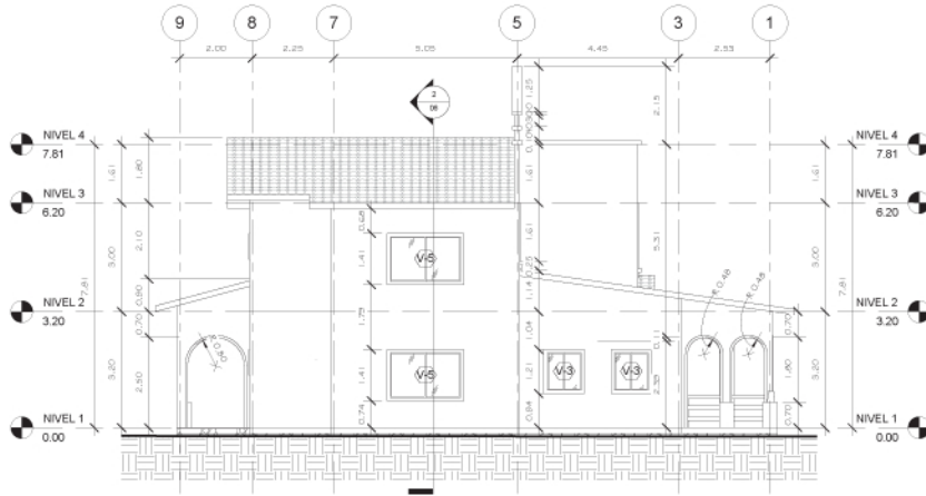
ELEVACION LATERAL IZQUIERDA
