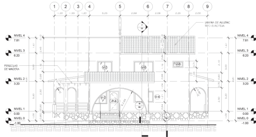
ELEVACION LATERAL DERECHA
