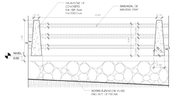
DETALLE DE BARANDAL Y BALAUSTRATE
