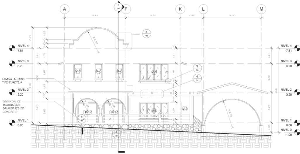
ELEVACION FRONTAL
