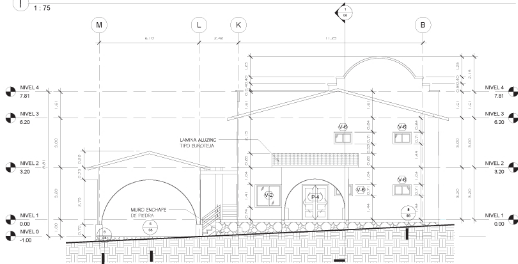
ELEVACION POSTERIOR
