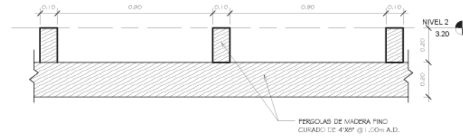
DETALLE DE PERGOLAS
