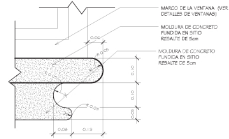
DETALLE DE MOLDURA EN VENTANA
