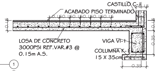
SECCION DE LOSA MONOLITICA 1:10
