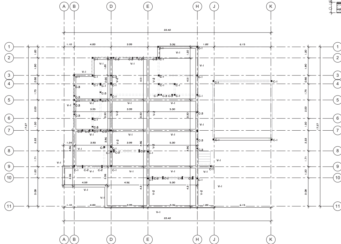
1 PLANTA ESTRUCTURAL DEL ENTREPISO 1:75
