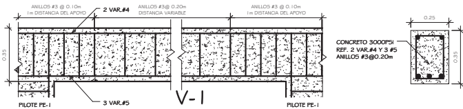
1:10 DETALLES DE VIGAS
