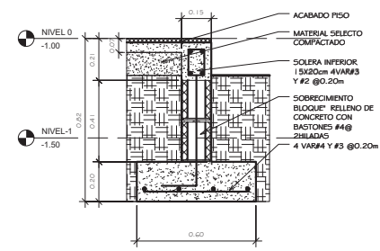
DETALLE DE CIMENTO CORRIDO
