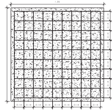
SECCION EN PLANTA DE ZAPATA Z-1
