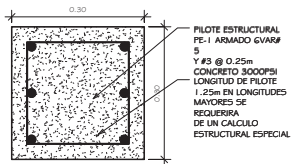
PILOTE ESTRUCTURAL PE-1 1:7.5
