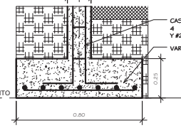
SECCION EN ALZADO DE ZAPATA Z-3
