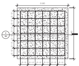
SECCION EN PLANTA DE ZAPATA Z-3
