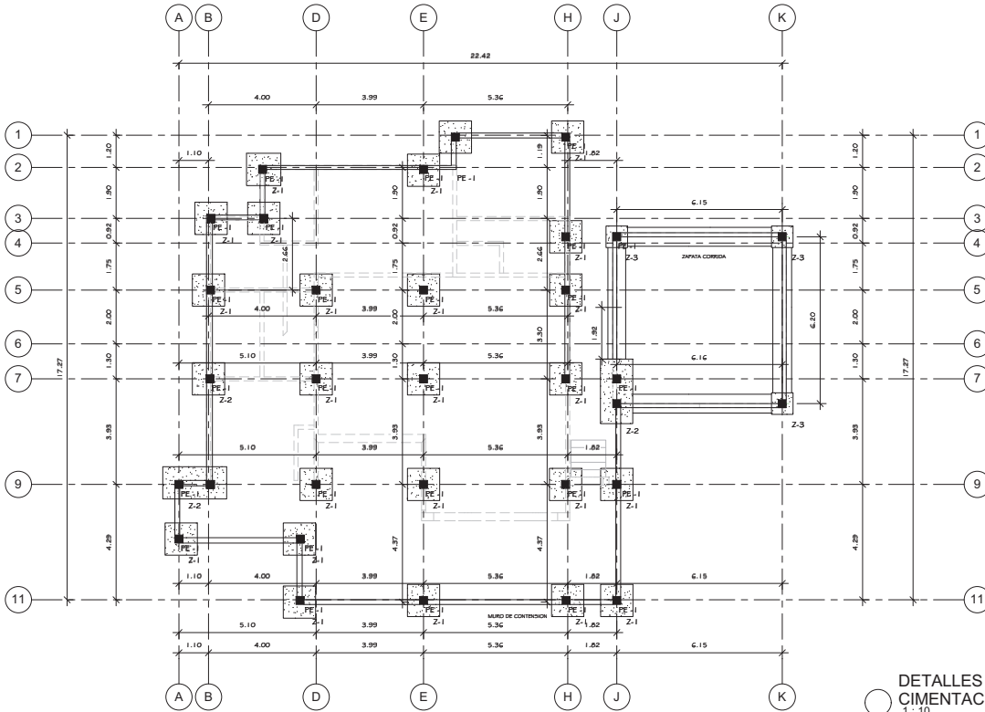
1 PLANTA ESTRUCTURAL DE CIMENTACION 1:7.5
