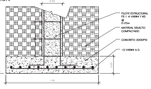
SECCION EN ALZADO DE ZAPATA Z-1
